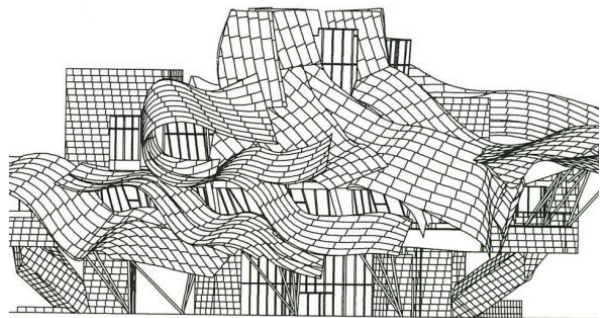
FIG. 7.7 Model en ontwerp-tekening hotel Marques de Riscal, Spanje [ref Frank Gehry, architect, 2001, Guggenheim Museum New York ISBN 0-89207-245-6]
